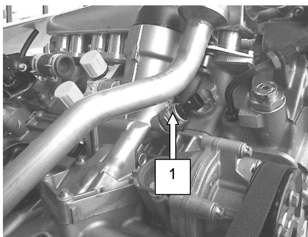
Bild / Figure 1 Einbaulage Öldrucksensor / Position Oil Pressure Sensor
